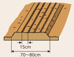
図3 トンネルの被覆
